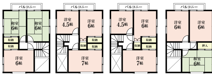
【2階間取り図】
